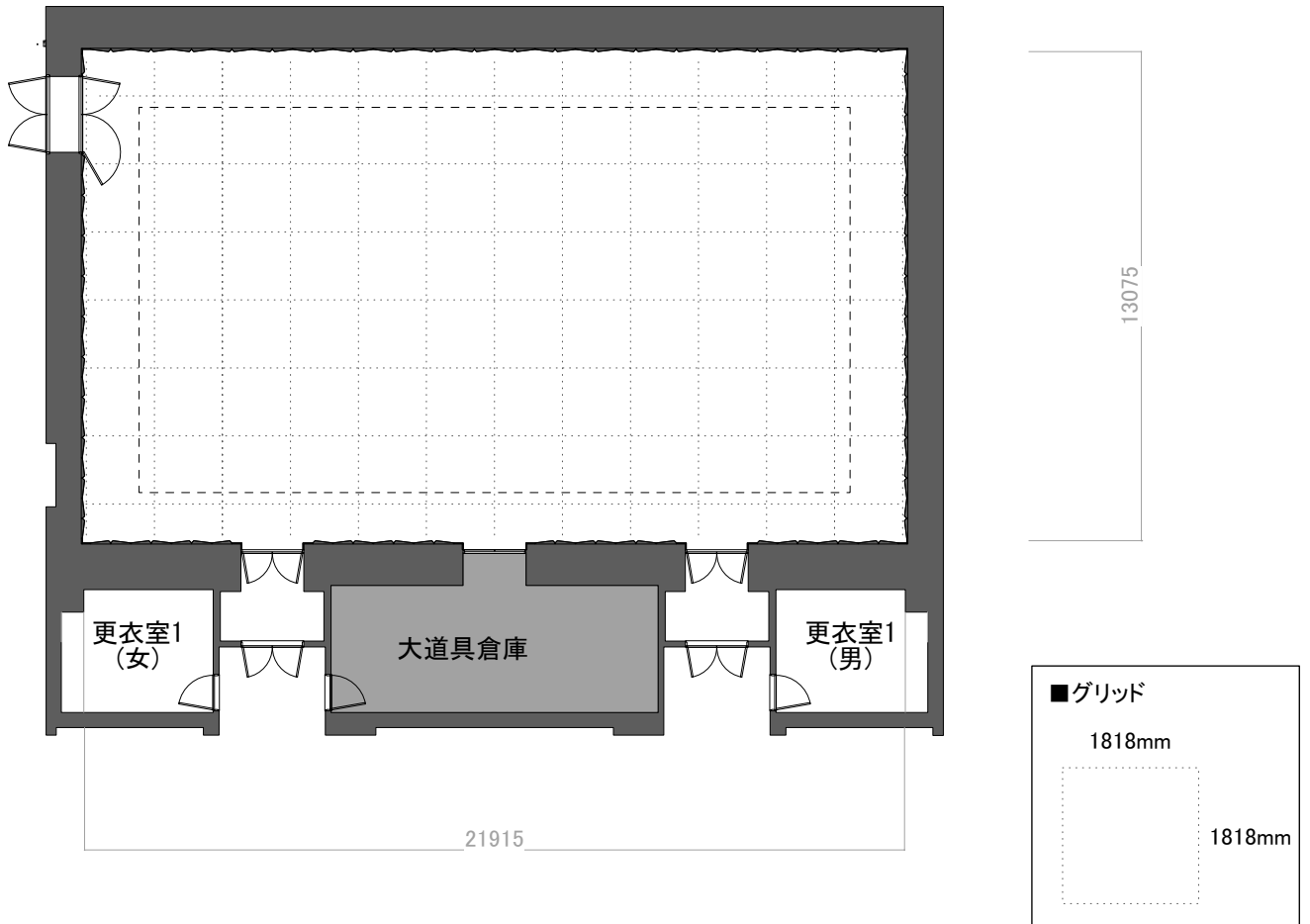
1階平面図
